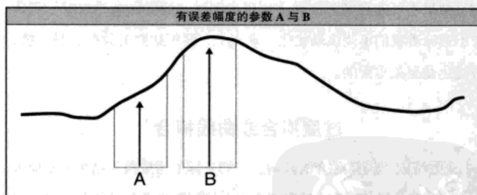
图 11-5 有误差幅度的参数 A 与 B
