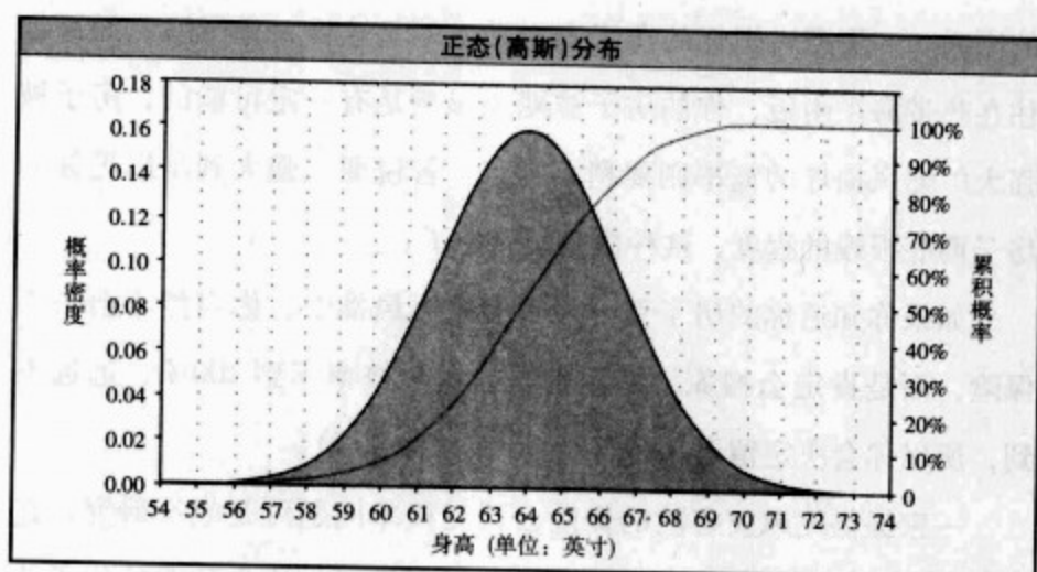
图 4-1 女性身高的概率分布
