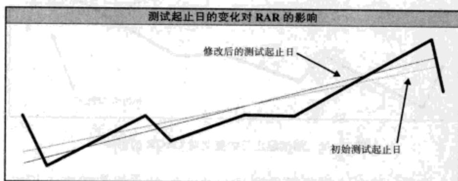
图 12-2 测试起止日的变化对 RAR 的影响
