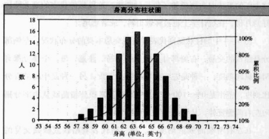
图 4-2 女性身高的柱状分布图
